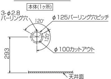
新鮮外気取入口詳細図
