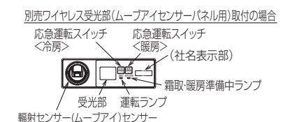
ムーブアイセンサーパネルの場合 (社名表示部)
