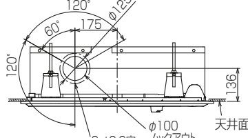
左側面 新鮮外気取入口詳細図
