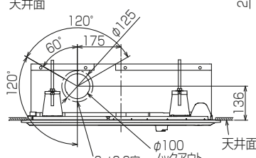
左側面 新鮮外気取入口詳細図
