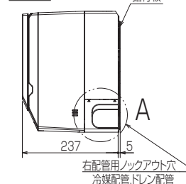
右側面図
