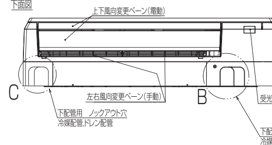
下面图
