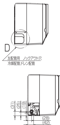
左側面図
