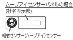
別売ワイヤレス受光部(ムーブアイセンサーパネル用)取付の場合 応急運転スイッチ <暖房> (社名表示部) 応急運転スイッチ <冷房> 霜取・暖房準備中ランプ 受光部 運転ランプ 輻射センサー(ムーブアイ)センサー
