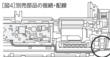
〔図4〕別売部品の接続・配線
