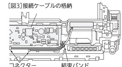
〔図3〕接続ケーブルの格納
