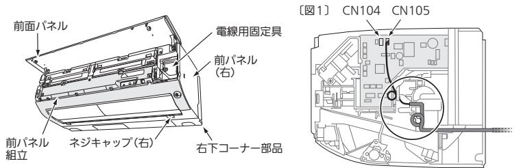
【図1】 CN104 CN105
