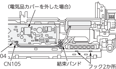
〈図1〉 室内制御基板
