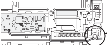
〈図4〉 別売部品の接続・配線
