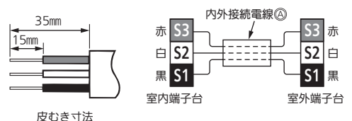
皮むき寸法
