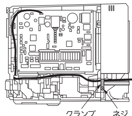
〈図3〉配線経路
