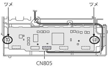
〈図2〉表示・ムーブアイ組立(裏面)
