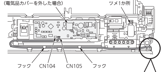
〈図2〉表示・ムーブアイ組立(裏面)
