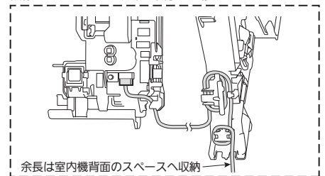
〈図1-1〉無線LANアダプターを取付ける場合
