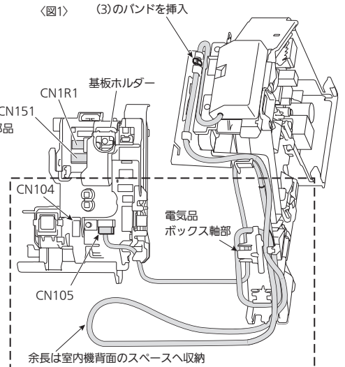
〈図1〉無線LANアダプター以外を取付ける場合
