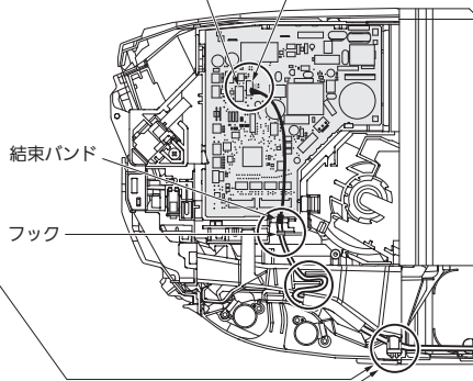
〈図1〉室内制御基板
