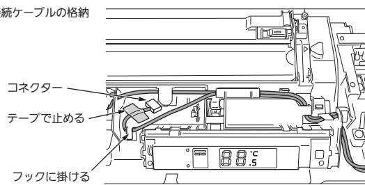
〈図2〉接続ケーブルの格納
