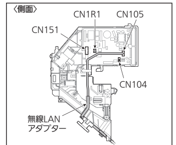
〈図1-1〉無線LANアダプター以外を取付ける場合
