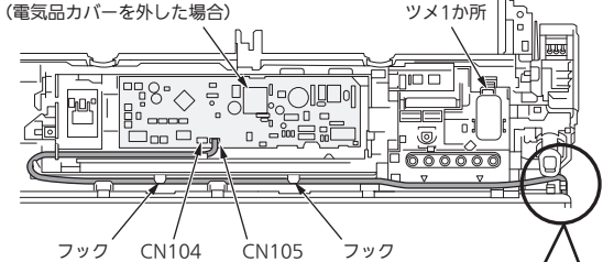
〈図2〉表示・ムーブアイ組立(裏面)
