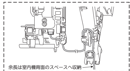
〈図1-1〉 無線LANアダプター以外を取付ける場合
