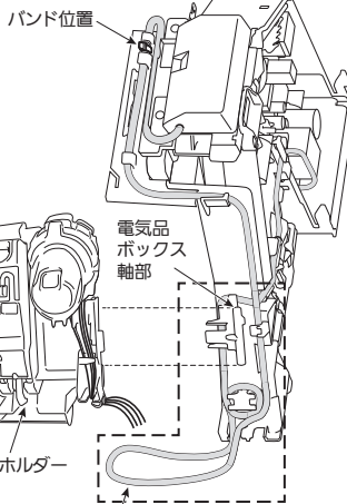
余長は室内機背面のスペースへ収納
