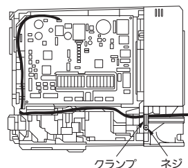
〈図3〉 配線経路
