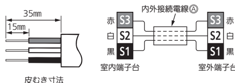
皮むき寸法
