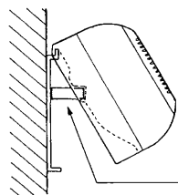
スペーサー
