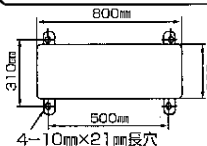
室外ユニット固定用穴位置図
