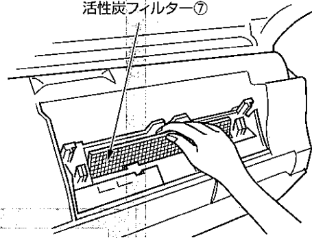
活性炭フィルター⑦
