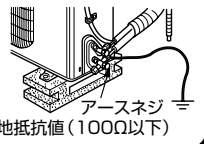
アースネジ 接地抵抗値(100Ω以下)
