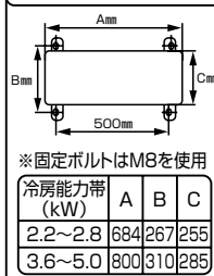
室外ユニット固定穴位置図
