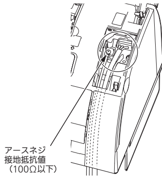
アース線(φ1.6mmまたは断面積2mm 2 以上)は付属されていません。(現地手配)
