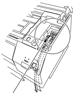
アースネジ 接地抵抗値 (100Ω以下)
