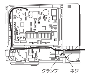
【図3】配線経路
