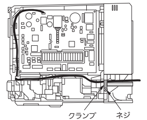
【図3】配線経路
