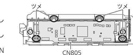
〔図4〕別売部品の接続・配線
