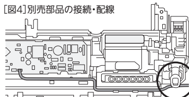
〔図4〕別売部品の接続・配線
