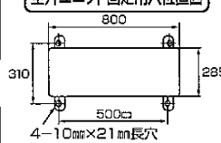
室外ユニット固定用穴位置図
