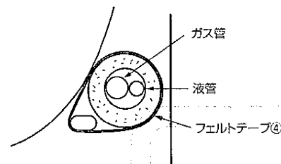
配管用穴
