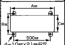
室外ユニット固定穴位置図
