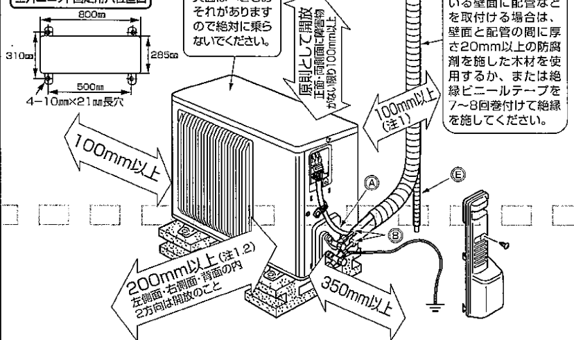
室外ユニット固定用穴位置図
