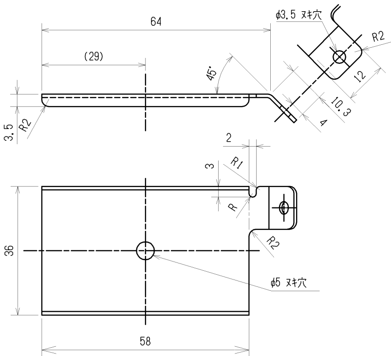
[リモコン取付具側金具]
