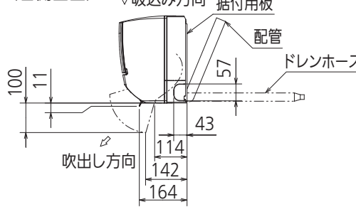
(右側面図)
