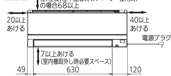
(正面図)
