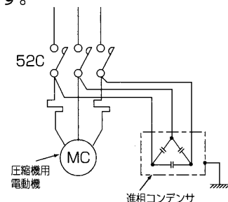
図9-1.進相コンデンサの接続
