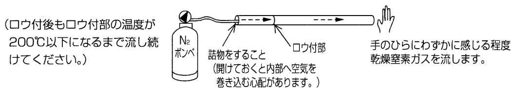
図6-2.無酸化ロウ付けの例
