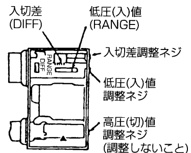
図10-1.高低圧圧力開閉器
