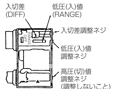
高低圧圧力開閉器
