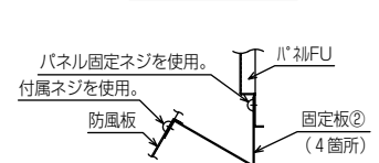
固定板②取付詳細図
