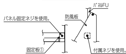
固定板①取付詳細図
