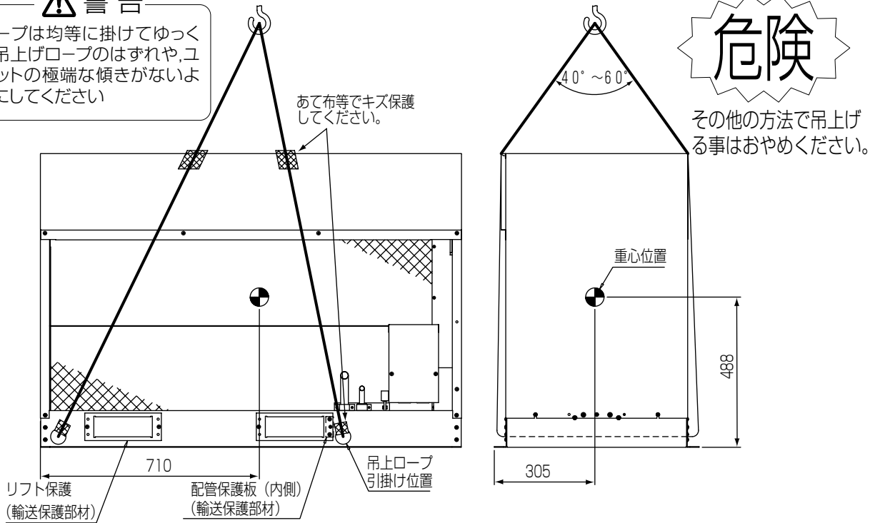
製品の吊下げ寸法
