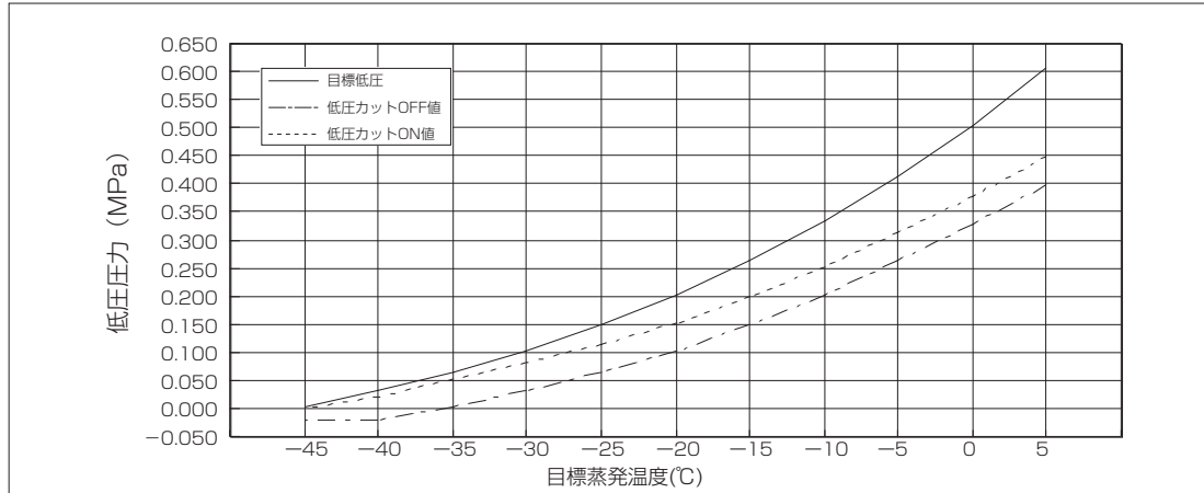
低圧相関図
