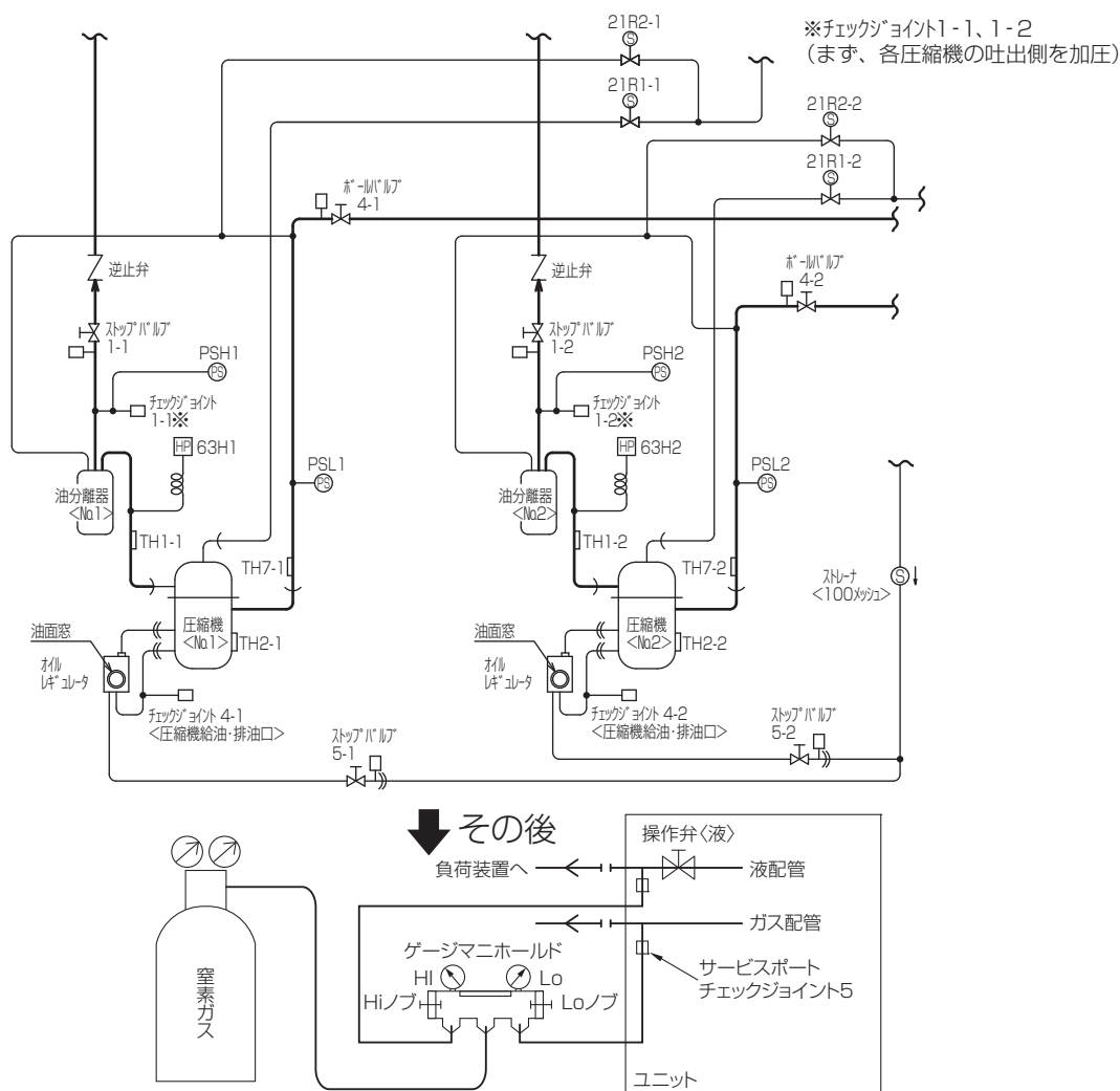
気密試験機器の接続系統図
