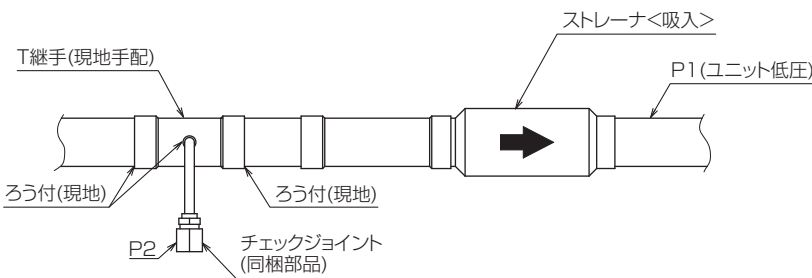
ストレーナ詰まりチェック用チェックジョイント
