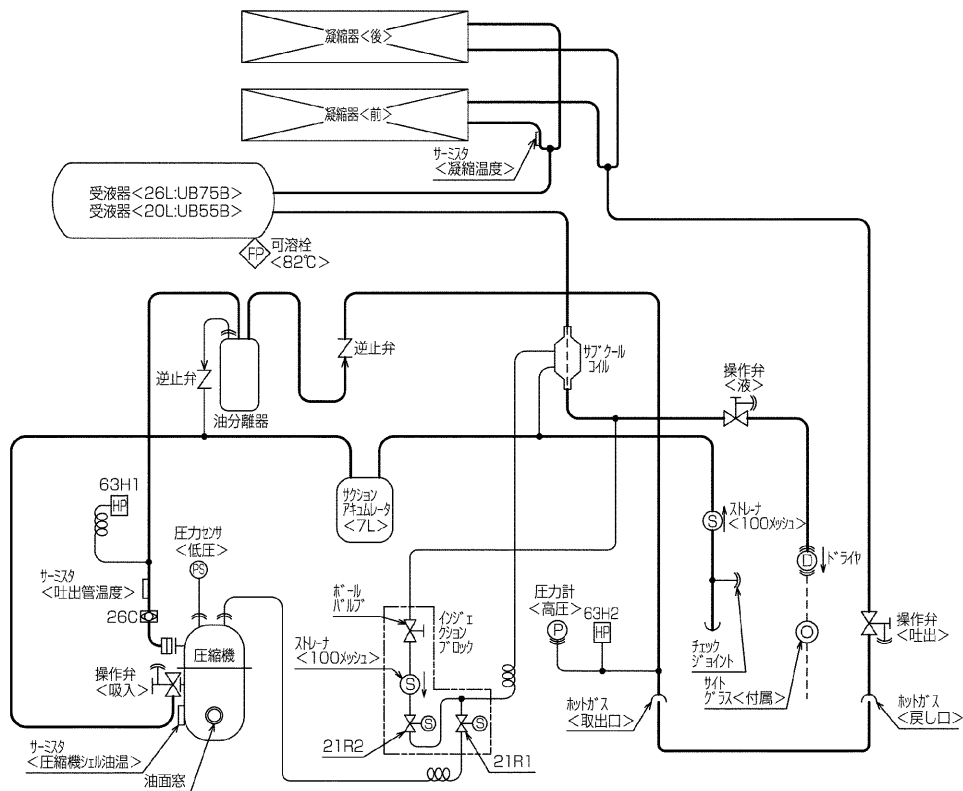
ERA-UB55B,UB75B 冷媒回路図と機器作動値
