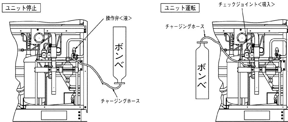
冷媒の充てん
