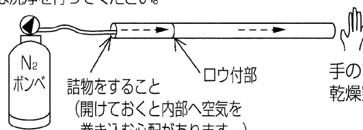
無酸化ロウ付けの例
