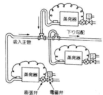
吸入配管
