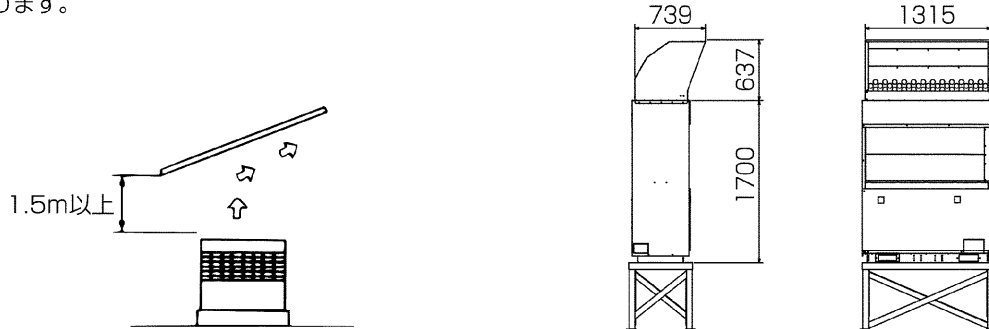
防雪フード取付け
