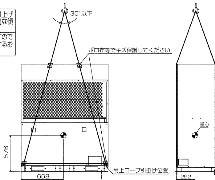
製品の吊下げ寸法
