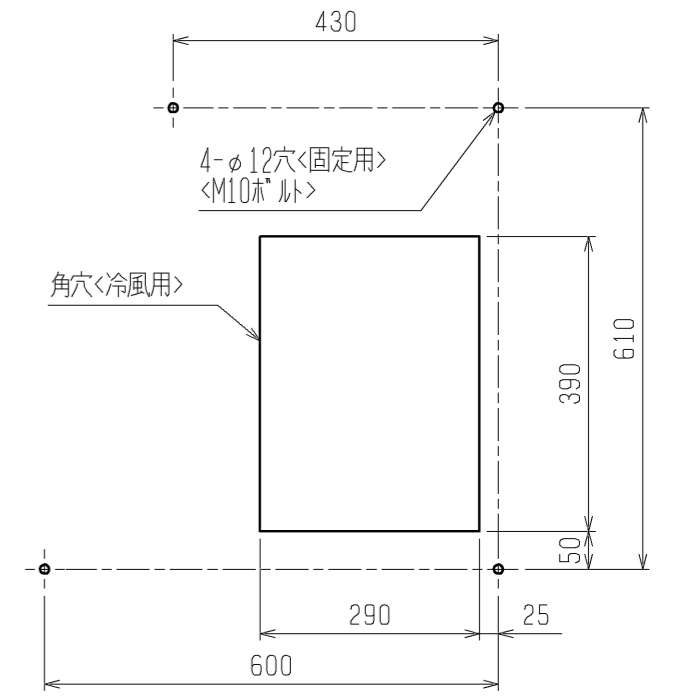
取付寸法
