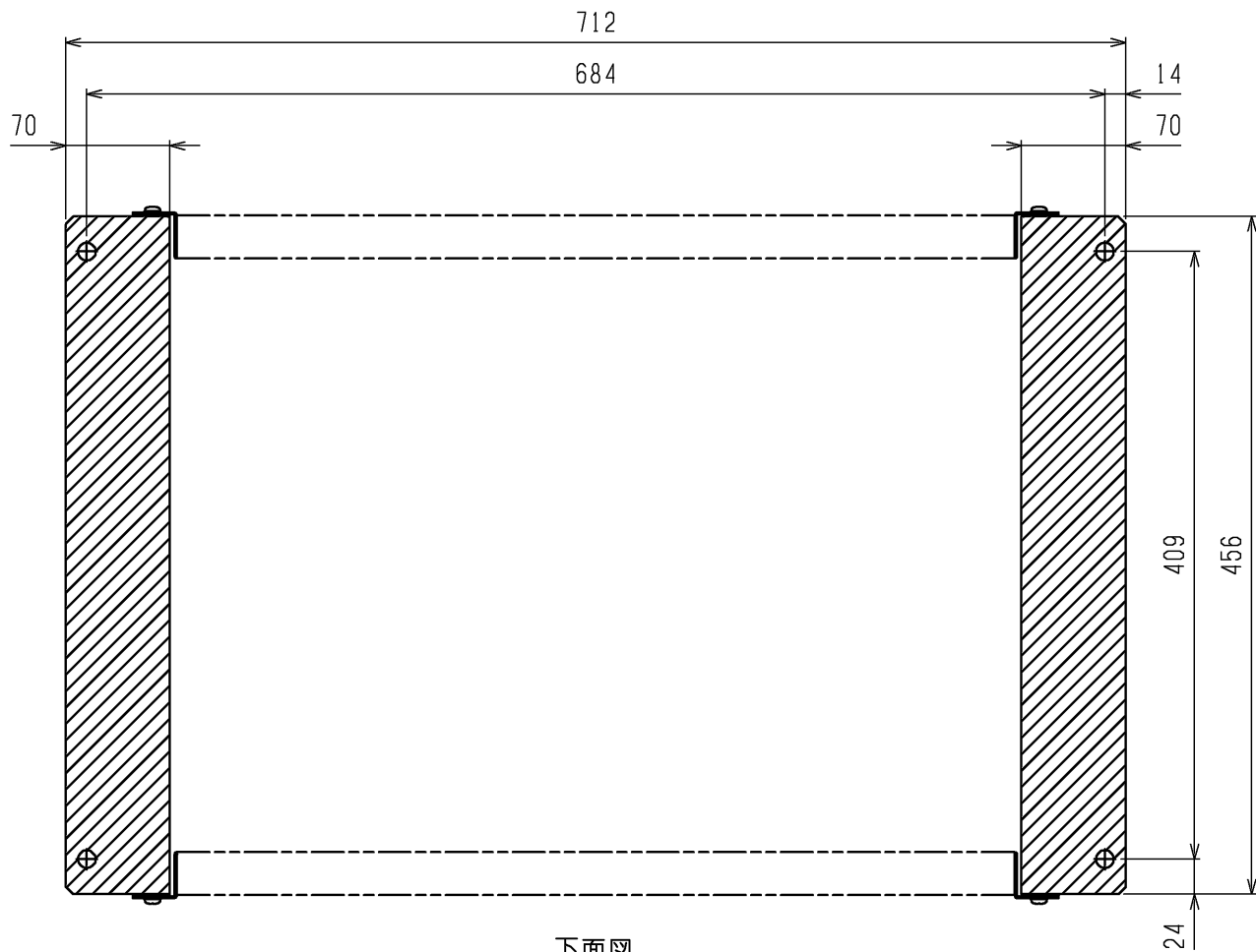
下面図
