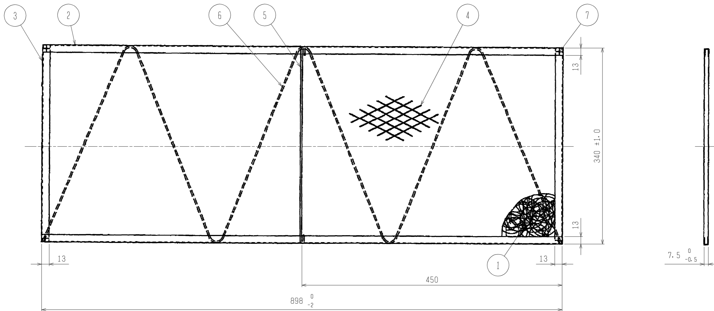
フィレドンフィルタ仕様表
