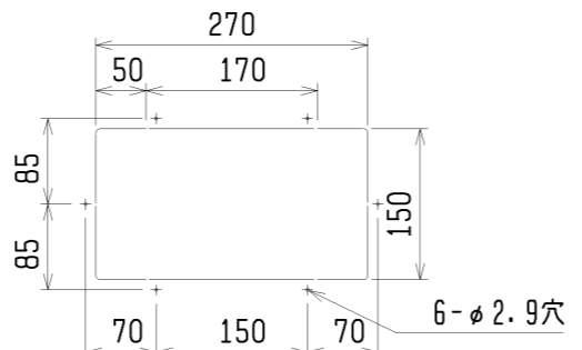
外気取込穴詳細図
