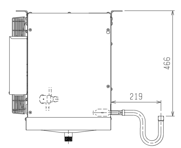
オイルラップ 取付時の寸法
