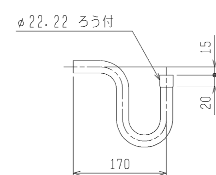
オイルラップ<付属>
