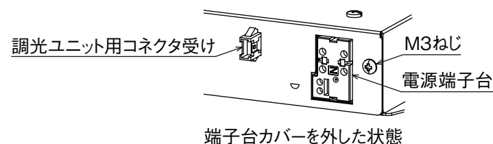
<上図はEL-GT40100N/Wを示す>
