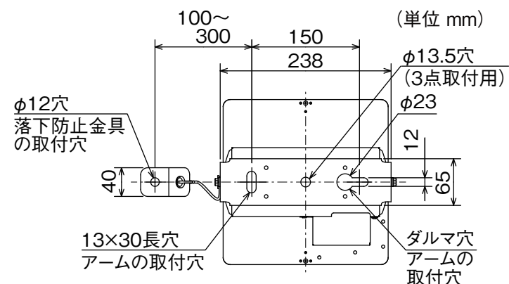
<上図はEL-GT20100N/Wを示す>
