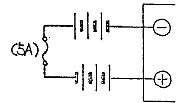
接続図
