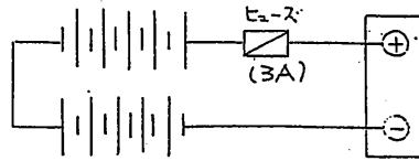
接続図
