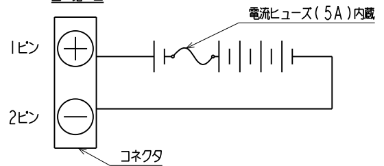
回路図
