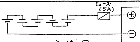
接続図
