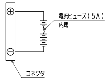
回路図
